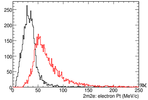
(d) Ordered p_T distributions of the 2 electrons in 2\mu 2e events.
